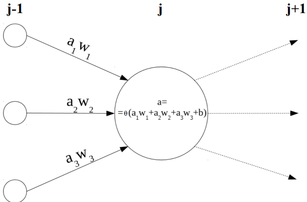
2 pav. Neurono, esančio sluoksnyje j , schema. Čia \theta - aktyvacijos funkcija, a - neurono aktyvacija, w - svoris, b - poslinkis.
