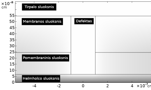
S.1 pav.: Trimačio tBLM membranos modelio schema. Kairėje: modelio skerspjūvis defekto aplinkoje. Dešinėje: šešiakampė prizmė, atitinkanti modeliavimo sritį.
