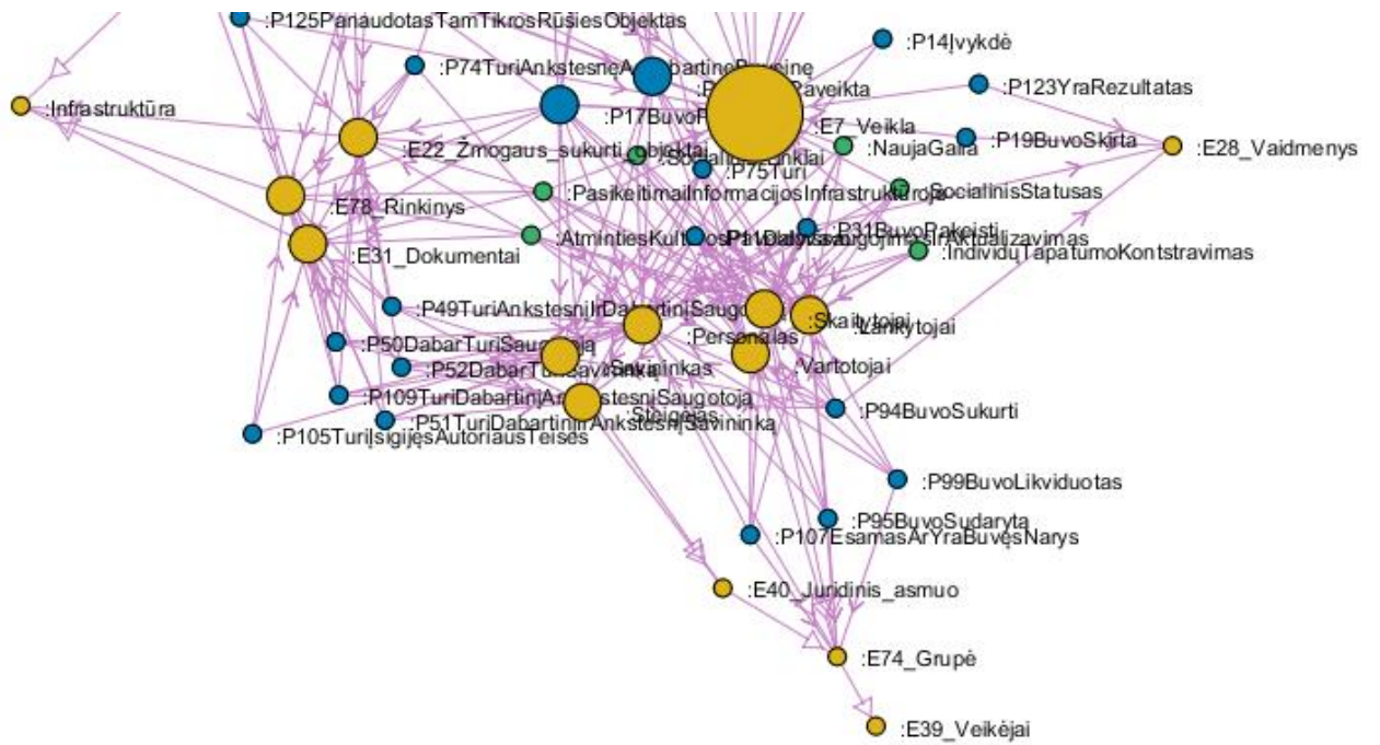
7 pav. Bibliotekų vaidmenų sąveika su bibliotekos sistemos esiniais
