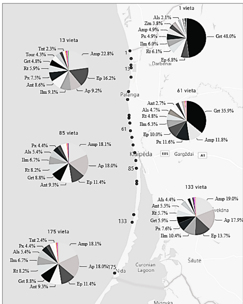
1 pav. Paplūdimio sąnašose aptinkamų sunkiųjų mineralų sandaigų sudėties pasiskirstymas Lietuvos pajūrio krante. Amp – amfibolai, Ap – apatitas, Als – aliuminio silikatai, Ant – anatazas, Ep – epidotai, Grt – granatai, Ilm – ilmenitas, Px – piroksenai, Tour – turmalinas, Tnt – titanitas, Rt – rutilas, Zrn – cirkonas.
