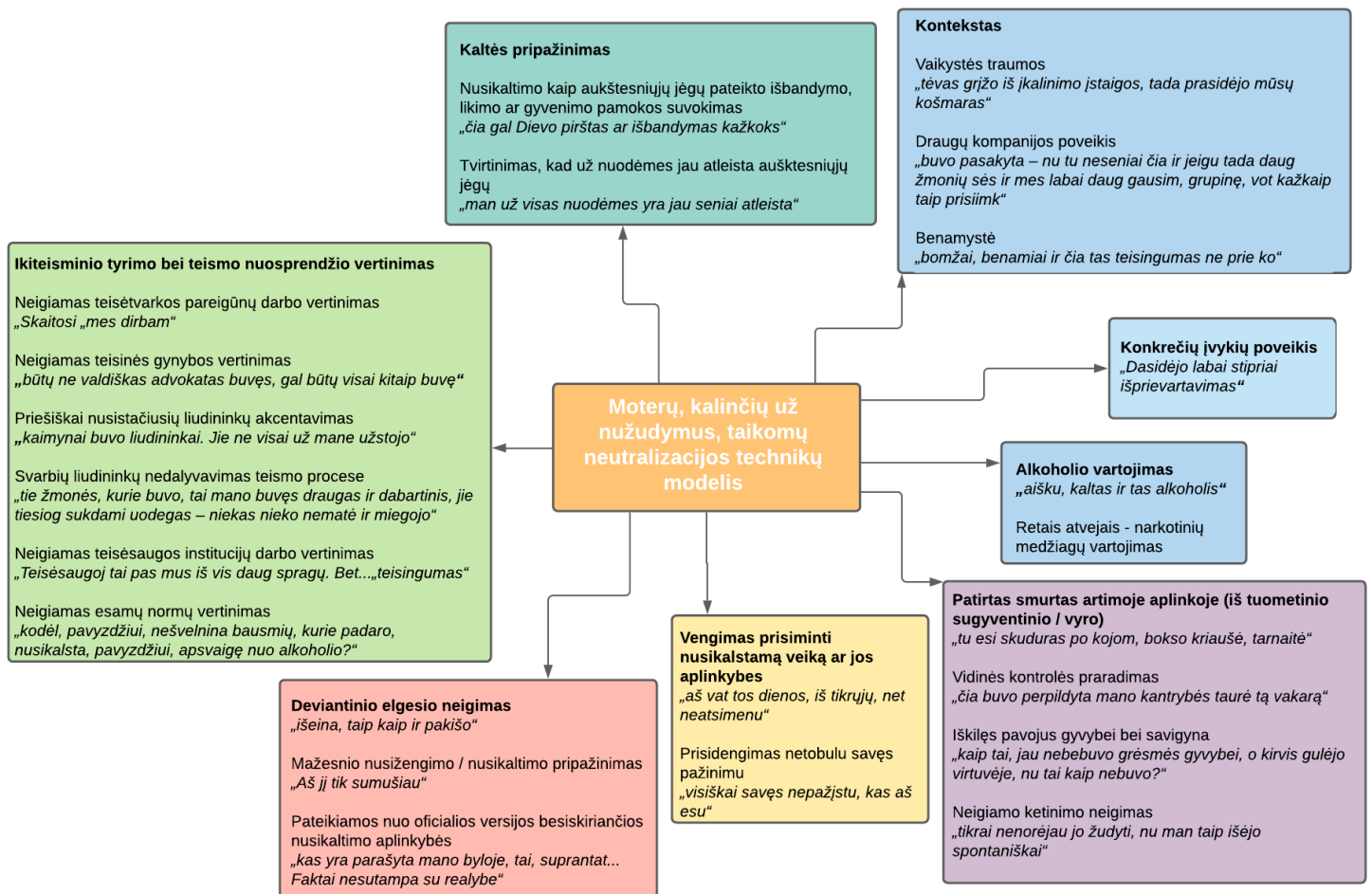
Diagrama Nr. 2: Moterų, atliekančių laisvės atėmimo bausmę už nužudymus, taikomų neutralizacijos technikų modelis
