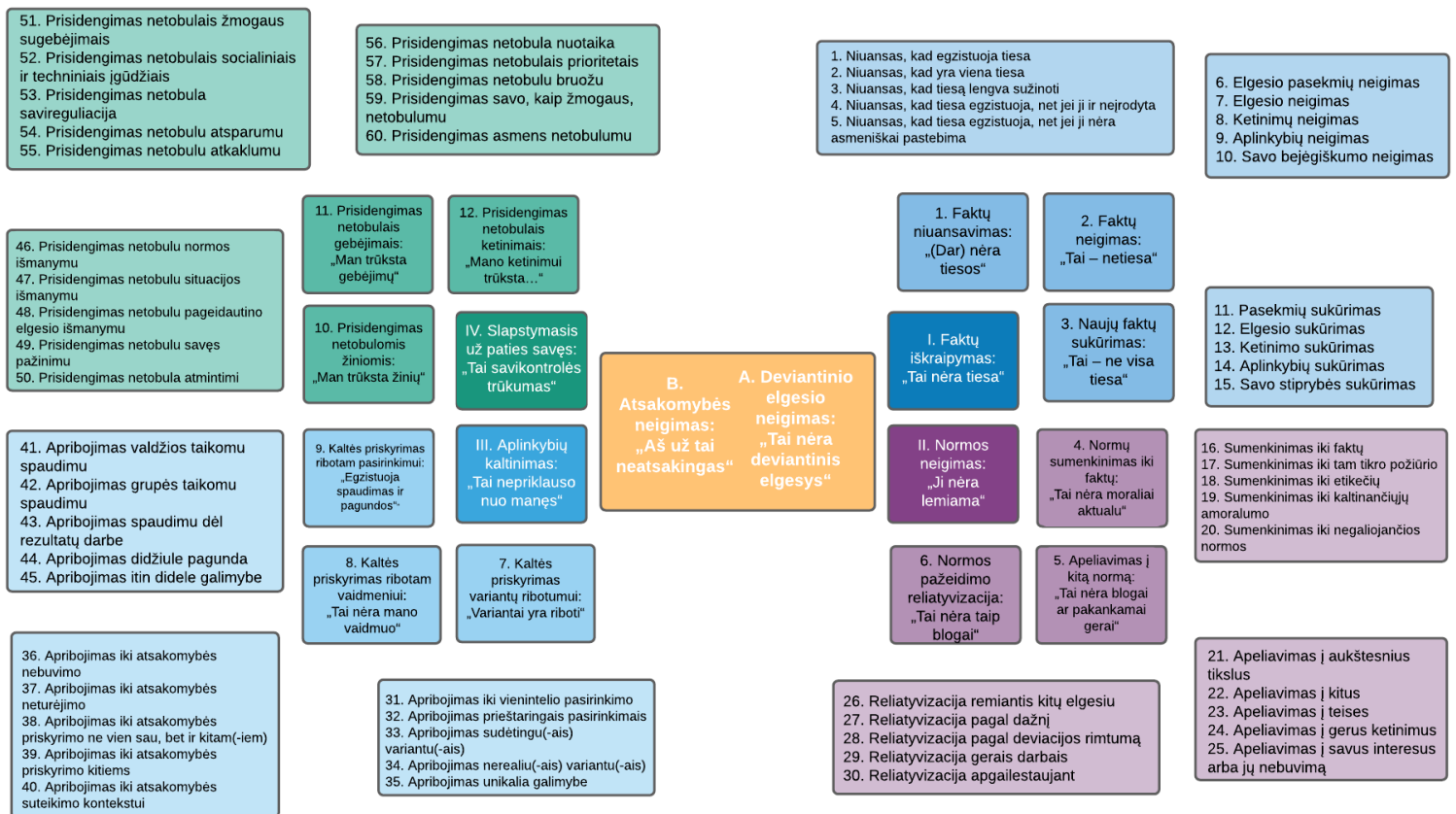
Diagrama Nr. 1: M. Kaptein ir M. van Helvoort susistemintas neutralizacijos technikų modelis
