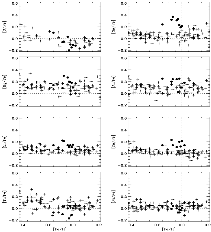
12 pav. Cheminių elementų gausa padrikojo spiečiaus NGC 7789 žvaigždžių atmosferose.
