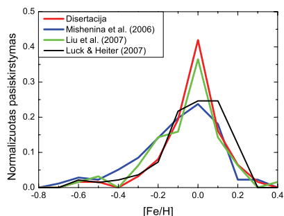
7 pav. Galaktikos sankaupos žvaigždžių metalingumo pasiskirstymo palyginimas pagal skirtingus autorius.
