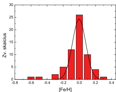
6 pav. Disertacijoje ištirtų Galaktikos sankaupos žvaigždžių pasiskirstymas pagal [Fe/H] . Juoda ištisinė linija pažymėta Gauso aproksimacijos funkcija.
