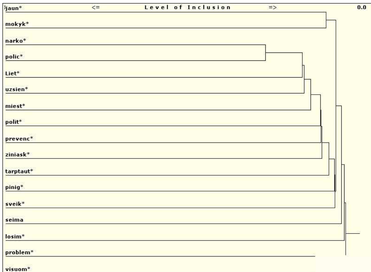
4 pav. „DELFI“ publikacijų narkotikų tematika klasterinė analizė 2000 m.
