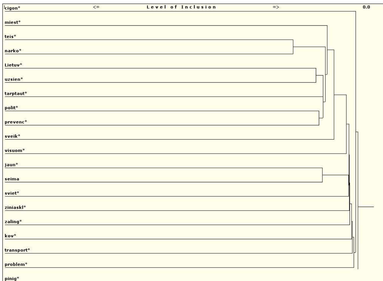
5 pav. „DELFI“ publikacijų narkotikų tematika klasterinė analizė 2005 m.
