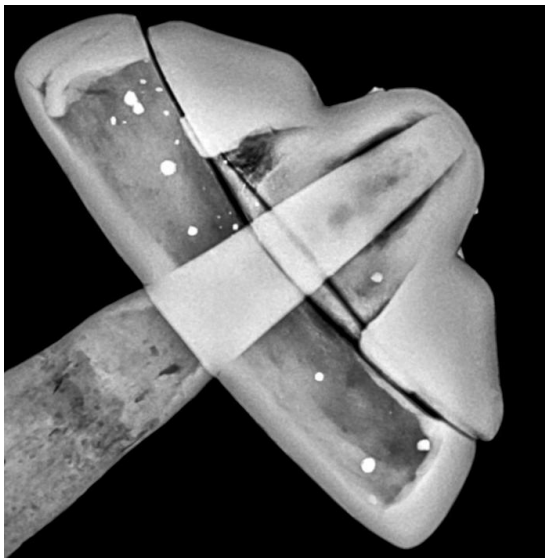
pav. 55. Paalksnių, Kelmės raj. kalavijo rankenos viršutinės dalies rentgenograma. Rentgenogramos autorius R. Vedrickas.
