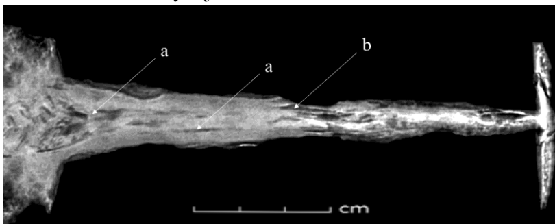
pav. 8. Taurapilio kalavijo (LNM AR 540:16) rentgenogramoje matomos gamybos žymės įklotėje. a – raštuoto plieno įvirinimas ir juostų suvirinimo siūlės, b – po apdirbimo natūraliai atsisluoksniavusios metalo juostos.
