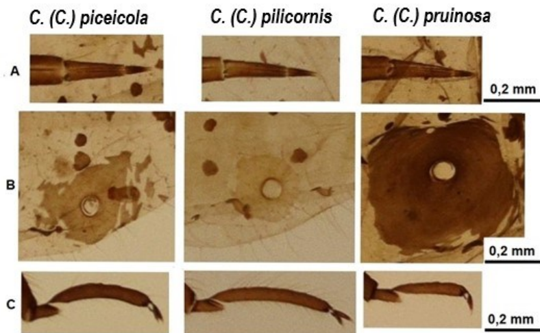
44 pav. Struktūros, su kuriomis susiję požymiai, leidžia Cinara ( Cinara ) pruinosa besparnes viviparas atskirti nuo C. (C.) piceicola ir C. (C.) pilicornis . A – R_IV+V. B – sifonas. C – užpakalinės kojos letenėlė. A. Petrašiūno nuotr.
