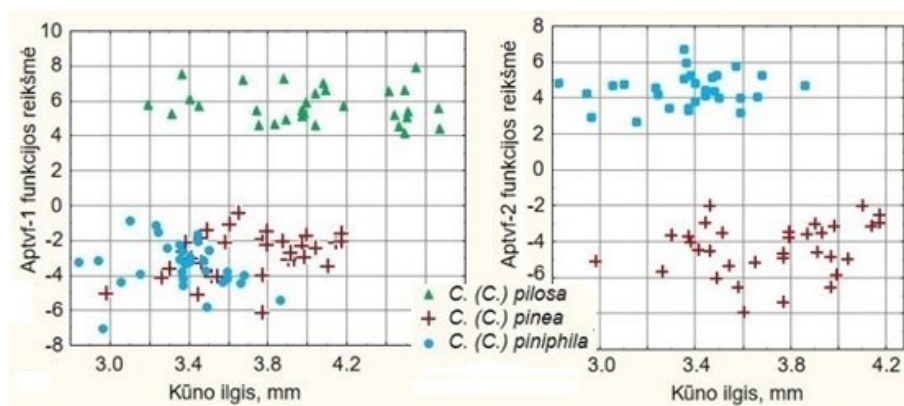
17 pav. Kanoninių funkcijų Aptvf-1 ir Aptvf-2, skirtų Cinara ( Cinara ) pilosa , C. (C.) pinea ir C. (C.) piniphila besparnėms viviparoms atskirti, reikšmės.
