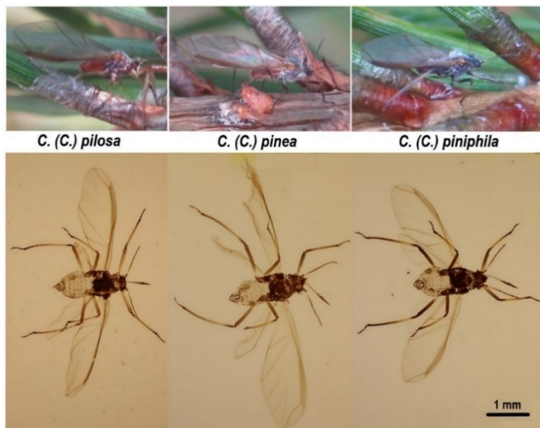
20 pav. Cinara (Cinara) pilosa , C. (C.) pinea ir C. (C.) piniphila patinai: viršuje – gyvi (J. Danilovo nuotr.); apačioje – preparuoti (A. Petrašiūno nuotr.)
