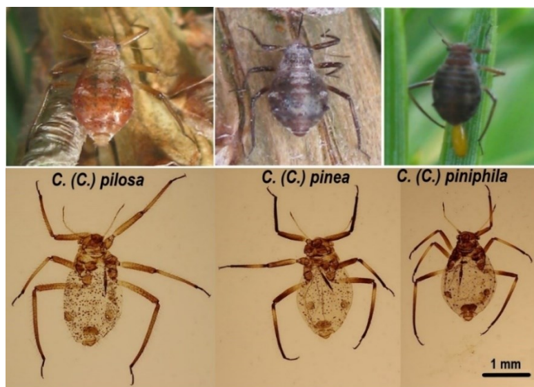
18 pav. Cinara ( Cinara ) pilosa , C. (C.) pinea ir C. (C.) piniphila oviparos: viršuje – gyvos (J. Danilovo nuotr.); apačioje – paruoštos (A. Petrašiūno nuotr.)
