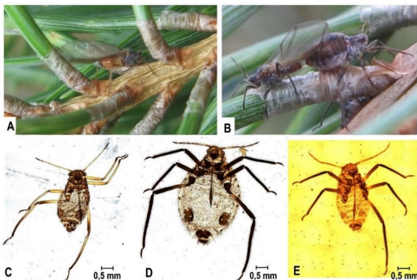
41 pav. Šio tyrimo metu pirmąkart registruotos amarų morfos. A – Cinara (Cinara) pilosa patinas; B – C. (Cinara) piniphila patinas (kairėje) ir ovipara (dešinėje); C – C. (Cinara) brauni besparnis patinas; D ir E – C. (Cupressobium) smolandiae : D – ovipara; E – patinas. J. Danilovo nuotr.
