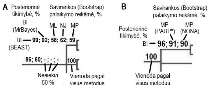
8 pav. Filogenetinio medžio fragmentų pavyzdžiai su paaiškinimais. A – pagal DNR sekas; B – pagal morfologinius ir biologinius požymius.
