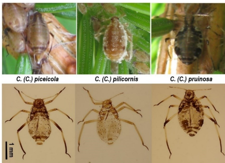
25 pav. Cinara (Cinara) piceicola , C. (C.) pilicornis ir C. (C.) pruinosa besparnės viviparos: viršuje – gyvos (J. Danilovo nuotr.); apačioje – paruoštos (A. Petrašiūno nuotr.)
