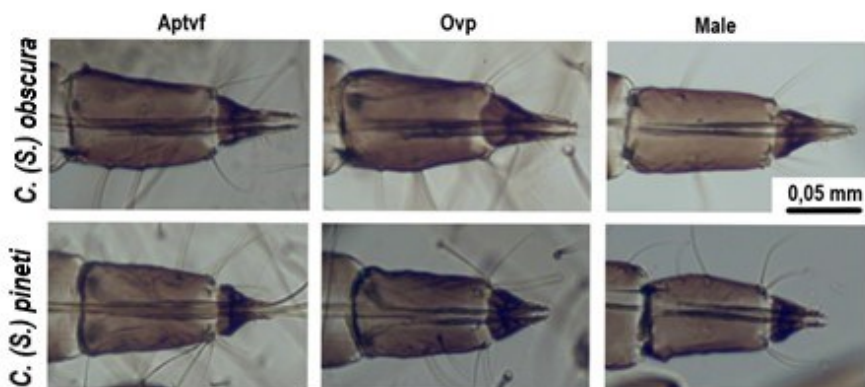
31 pav. Cinara (Schizolachnus) obscura ir C. (S.) pineti R_IV ir R_V. Amarų morfos: Aptvf – besparnės viviparos; Ovp – oviparos; Male – patinai.
