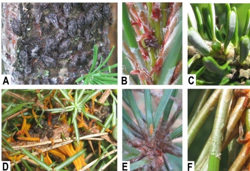
9 pav. Lietuvoje pirmąkart aptiktos Eulachnini tribos amarų rūšys.
