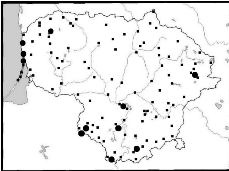
7 pav. Vietos, kur 2016–2020 m. rinkti amarai (kvadratai) ir vykdyti periodiniai amarų stebėjimai (skrituliai).
