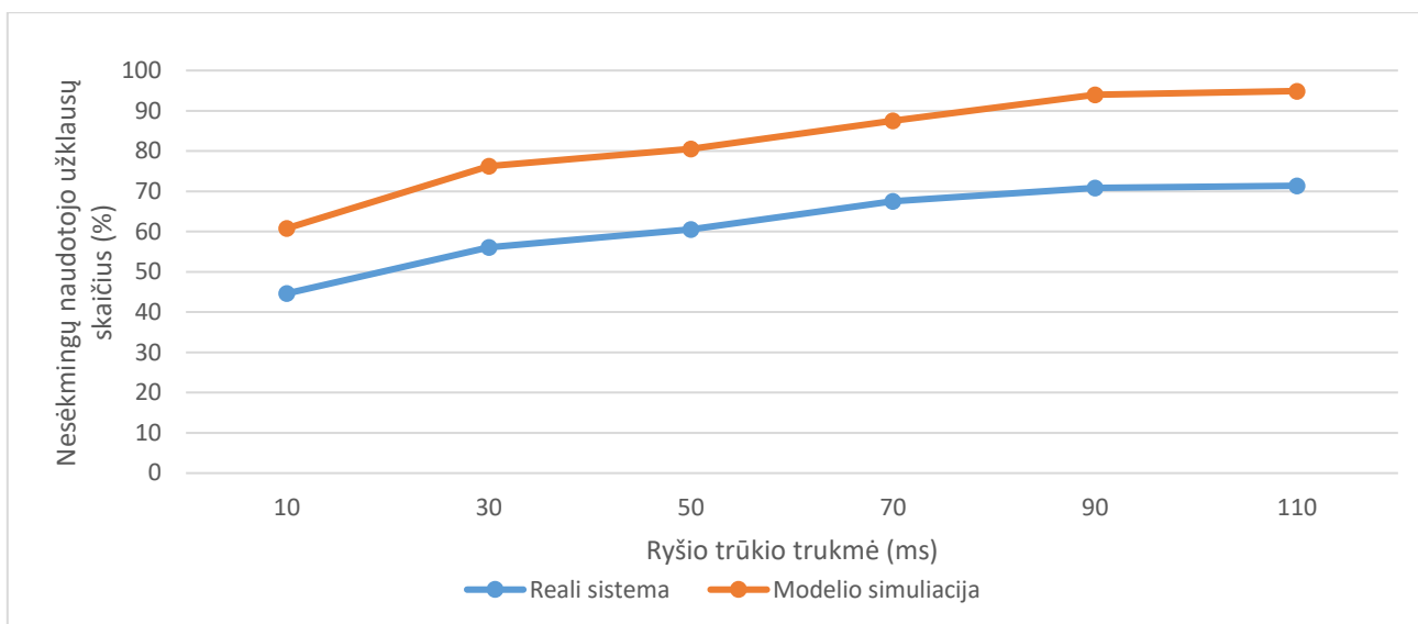
6 pav.: Nesėkmingų naudotojo užklausų skaičius procentais priklausomai nuo ryšio trūkio trukmės diagrama.
