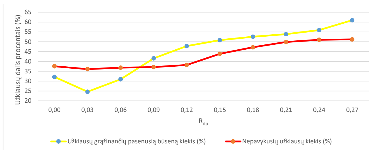
14 pav.: Užklausų grąžinančių pasenusią būseną kiekio priklausomybė nuo ryšio patikimumo kartu su nepavykusių užklausų kiekiu, kai naudotojo, kurio užklauskos nekeičia būsenos parametras V_{umax} = 2 .
