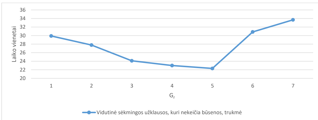
18 pav.: Sėkmingos užklauskos, kuri nekeičia būsenos, trukmės priklausomybė nuo dublikatų kiekio G_r .
