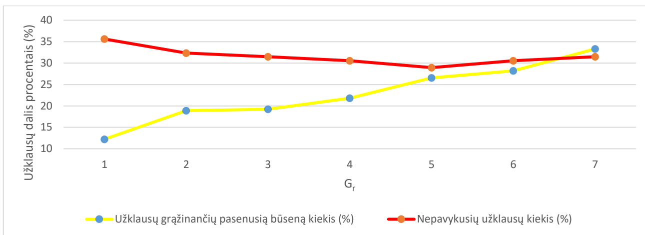
17 pav.: Užklausų grąžinančių pasenusią būseną kiekio bei nepavykusių užklausų kiekio priklausomybė nuo dublikatų kiekio G_r .
