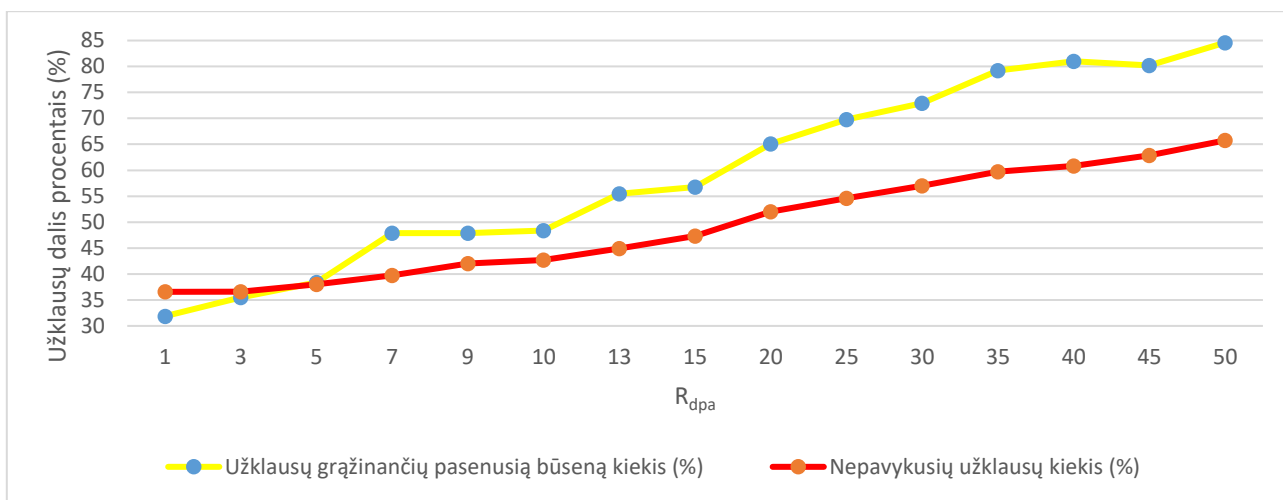
15 pav.: Užklausių grąžinančių pasenusią būseną kiekio priklausomybė nuo ryšio atstatomumo.
