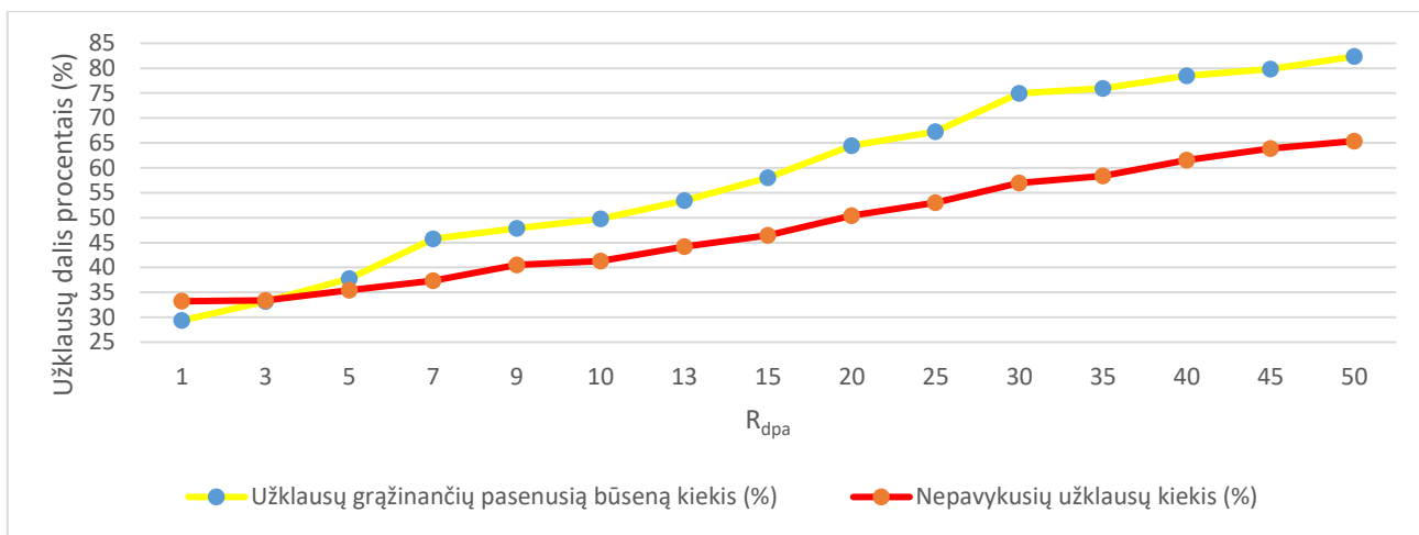
16 pav.: Užklausių grąžinančių pasenusią būseną kiekio priklausomybė nuo ryšio atstatomumo, kai naudotojo, kurio užklaustos nekeičia būsenos parametras V_{umax} = 2 .
