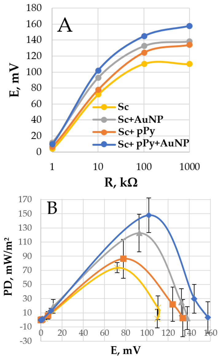
11 paveikslas. A. Potencialų priklausomybės nuo apkrovos. B. Galios tankio (PD) priklausomybės nuo potencialo. Matavimai atlikti PBS tirpale su gliukoze (20 mM) ir K_3 [Fe(CN)_6] (20 mM). Naudoti elektrodai buvo padengti PQ ir S. cerevisiae su įvairiais pakeitimais, parodytais 8 paveiksle.
