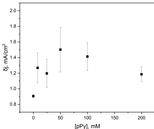
17 paveikslas. Diferencinio srovės tankio priklausomybė nuo pPy koncentracijos, naudojamos mielių ląstelių modifikavimui, naudojant PQ-pPy mielių-grafito elektrodo konstrukcijoje. Vertės buvo paimtos kaip \text{Fe}^{2+} oksidacinio piko \delta j vertės.
