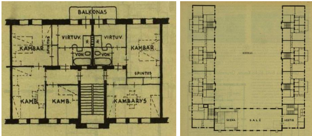
14 iliustracija. Griunvaldo g. darbininkų namo planai (St., „Darbininkų butų bloko Kaune, Griunvaldo g. projektas“, Savivaldybė , 1940, Nr. 7–8, p. 227–229).
