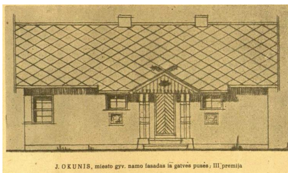
J. OKUNIS, miesto gyv. namo fasadas iš gatvės pusės, III premija
