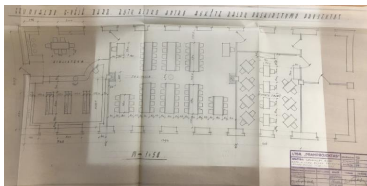
17 iliustracija. Griunvaldo gatvėje darbininkų butų bloko antro aukšto baldų paskirstymo projektas (VRVA, f. AKP, ap. 401/1–100, l. 81).
