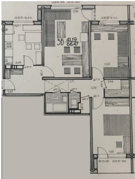
28 iliustracija. 3 kambarių buto planas pagal 1972 m. V. Krūminio ir V. Zubraus parengtą naują tipinių gyvenamųjų namų projektų seriją 120 V (VRVA, f. 1171, ap. ATD, b. 1160).
