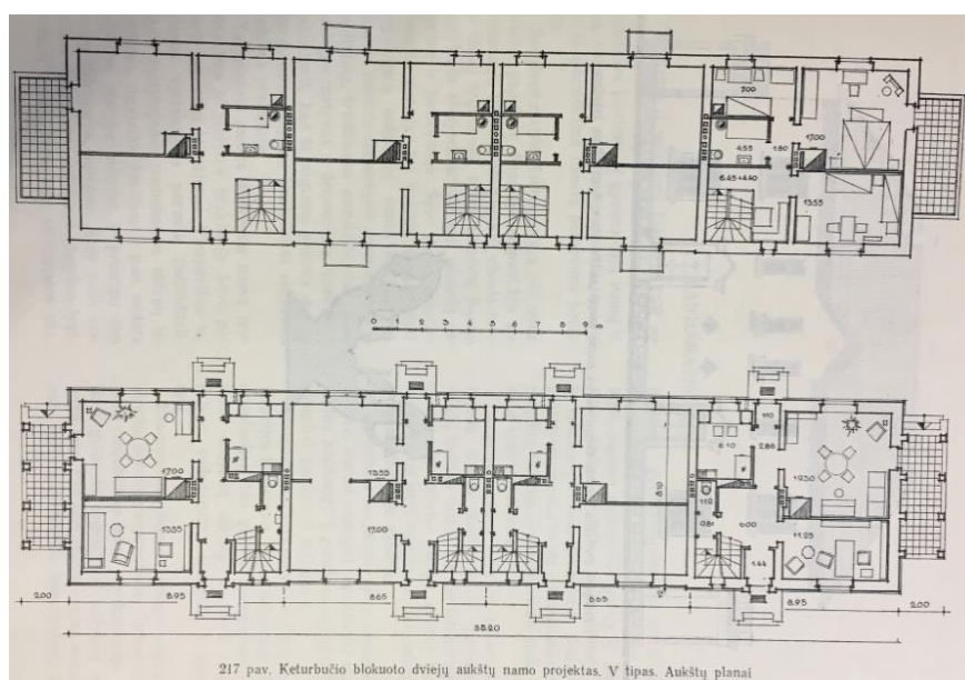
24 iliustracija. Keturbučio blokuoto dviejų aukštų namo projektas (Spelskis Antanas, Miestų sodybinės statybos architektūra , Vilnius, 1955, p. 209).
