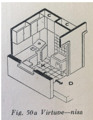
39 iliustracija. Virtuvė-niša (J. Okunis, Gyvenamieji namai , p. 71).
