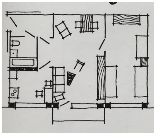
26 iliustracija. Serija 1-464LT, 2 kambarių butas (Витас Феликсас, Функциональное и пространственное решение интерьера современной квартиры Литовской ССР , in: LLMA, f. 772, ap. 1, b. 2, l. 115).
