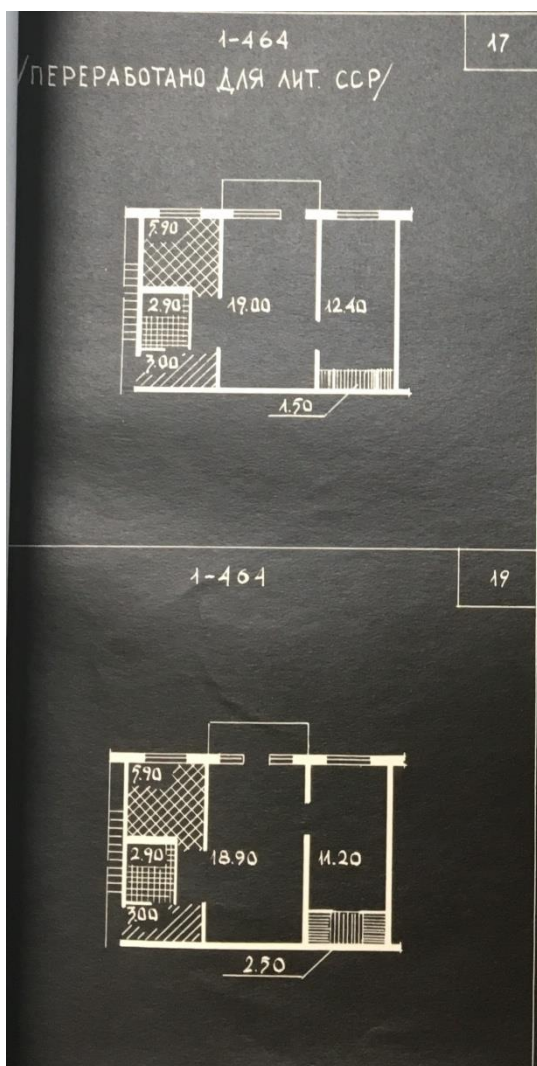
27 iliustracija. Serijos 1-464 buto planas po ir prieš adaptaciją statyboms Lietuvos TSR. Medžiaga iš miestų statybos projektavimo instituto mokslinės-techninės ataskaitos (VRVA, f. 1036, ap. 11, b. 236, l. 17).
