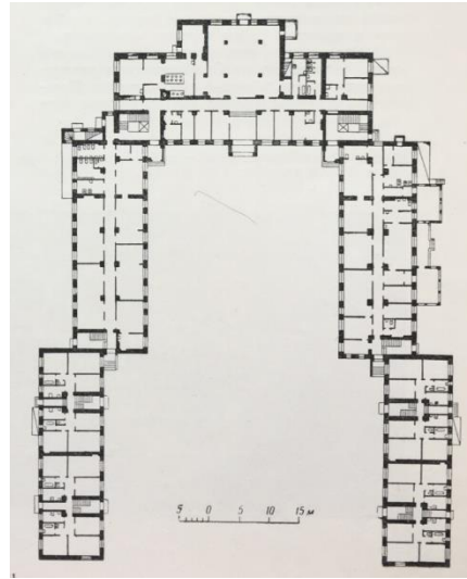
10 iliustracija. Namų-komunos projektas Maskvoje, Chavskoj g., 1928 m., arch. G. Volferzon, S. Leontovič, A. Barulin, ( Вопросы современной архитектуры , Maskva, 1962, Nr. 1, p. 9–69).
