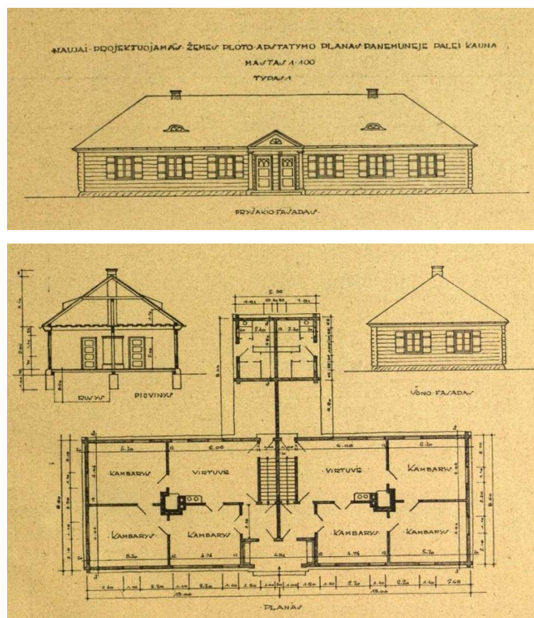
5 iliustracija. Vienas iš E. Peyerio pasiūlytų namų modelių – sublokuotas namas dviem šeimoms (Peyeris Eduardas, „Panemunės būstinės projektas“, Statybos menas ir technika , 1922, Nr. 2, p. 5).
