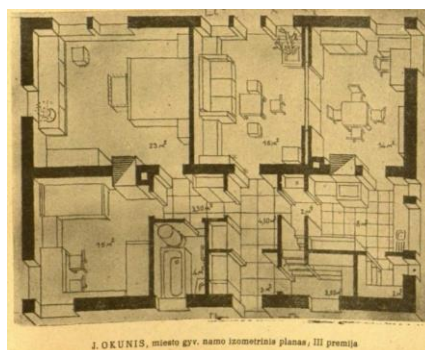
J. OKUNIS, miesto gyv. namo izometrinis planas, III premija
