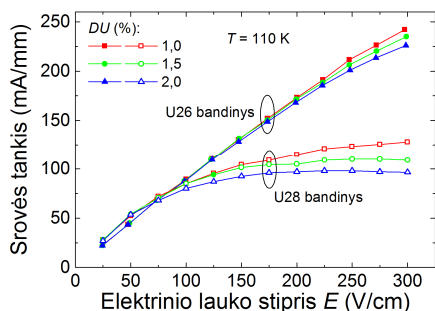
6.1 pav. U26 ir U28 bandiniais tekančios srovės tankio, gauto sunormavus srovę į bandinio plotį L , priklausomybė nuo elektrinio lauko stiprio 110 K temperatūroje esant skirtingoms DU vertėms [P2].
