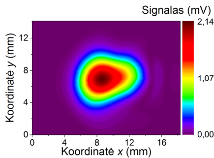
4.5 pav. 0,3 \text{ THz} dažnio spinduliuotės šaltinio sufokusuoto pluošto skerspjuvio atvaizdas, gautas naudojant U33 bandinio BT diodą, kurio sąsmaukos plotis 7 \mu\text{m} .
