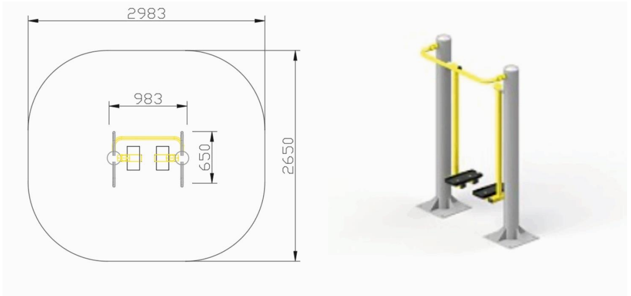
5pav. Lauko treniruoklis ir jo brėžinys
