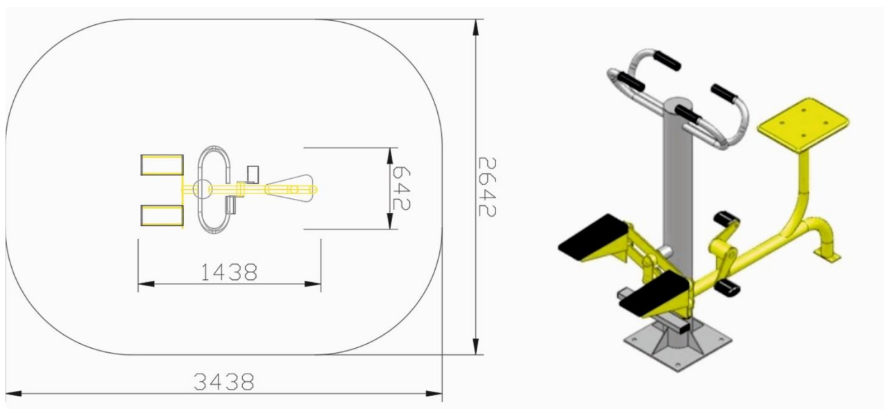
7pav. Lauko treniruoklis ir jo brėžinys
