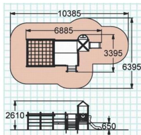
2pav. Žaidimų aikštelės brėžinys
