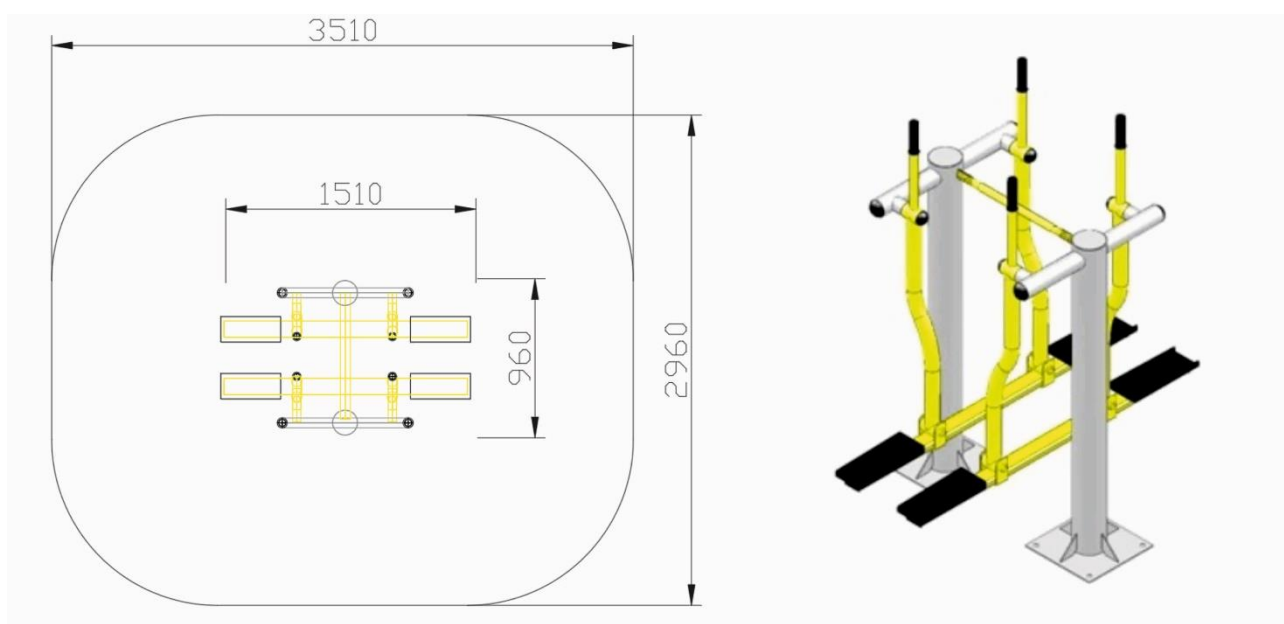
10pav. Lauko treniruoklis ir jo brėžinys
