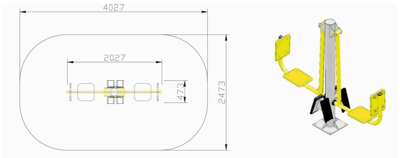
6pav. Lauko treniruoklis ir jo brėžinys
