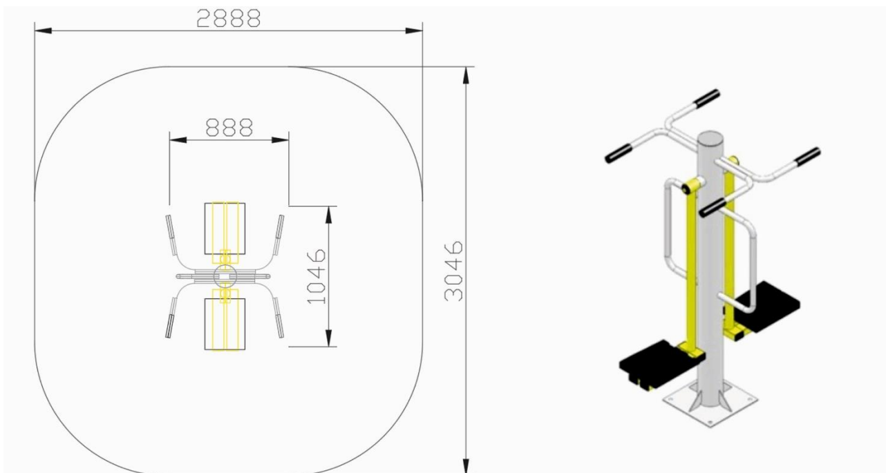
8pav. Lauko treniruoklis ir jo brėžinys
