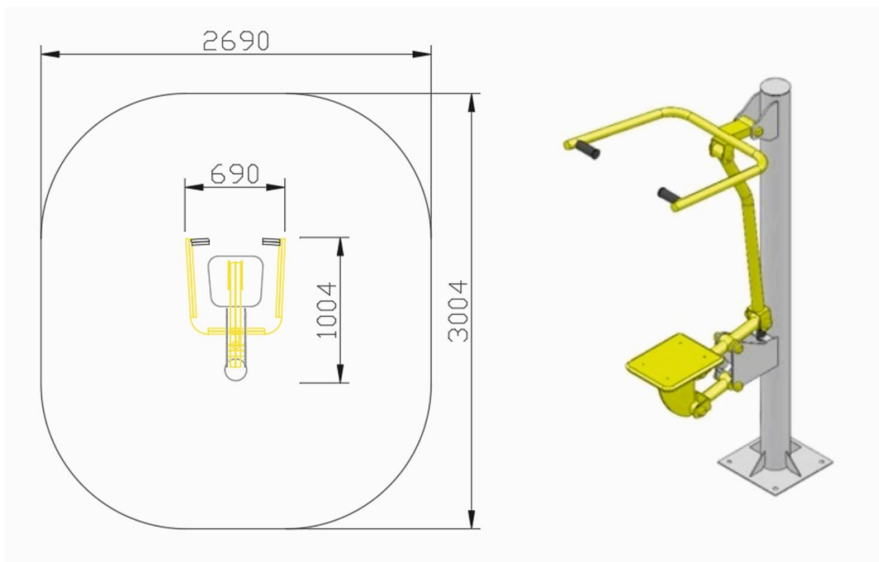
9pav. Lauko treniruoklis ir jo brėžinys
