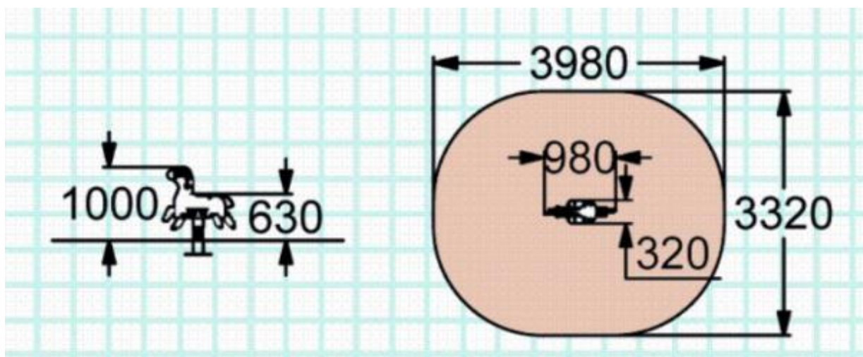
4 pav. Sūpynės su spyruokle brėžinys
