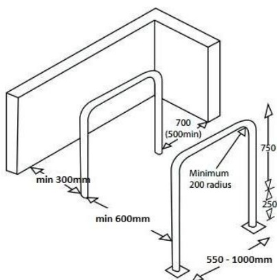
14 pav. Dviračio stovas ir jo brėžinys
