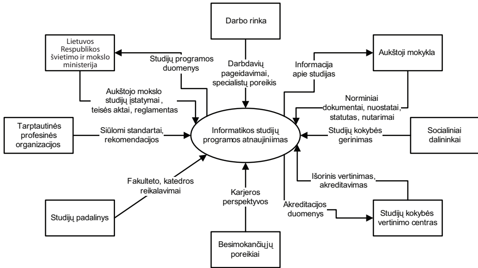
2 pav. Proceso „Informatikos studijų programos atnaujinimas“ konteksto modelis (aukščiausiojo lygmens TOP DFD)
