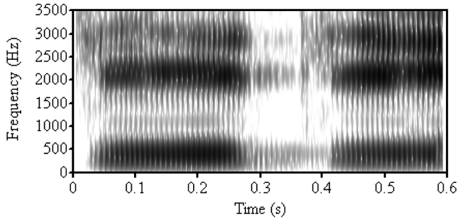
14 pav. Žodžio dėdė. ~ dėdė spektrograma
